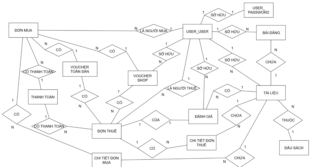
Hình 27: Lược đồ ERD văn tắt
