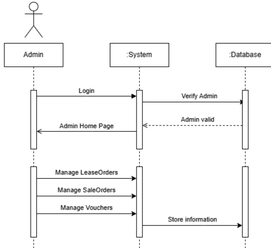
Hình 20: Sequence diagram cho quản trị viên
