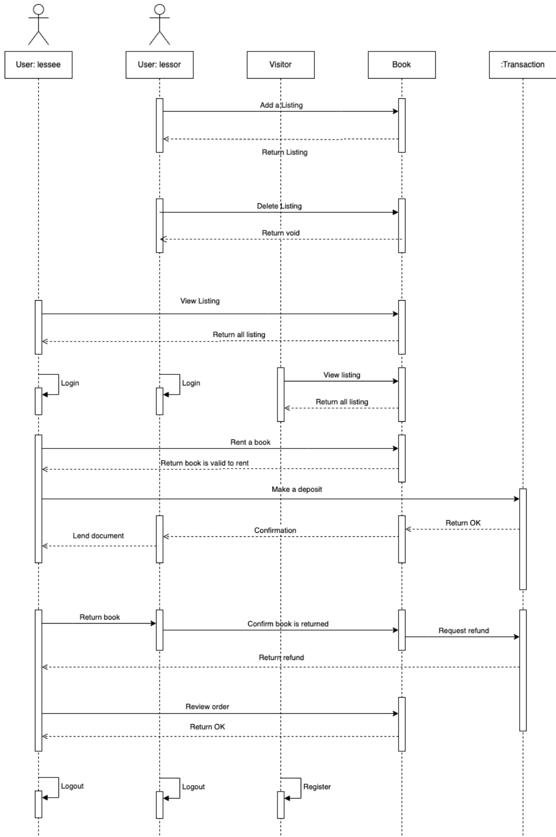
Hình 21: Sequence diagram cho người dùng và khách thuê sách
