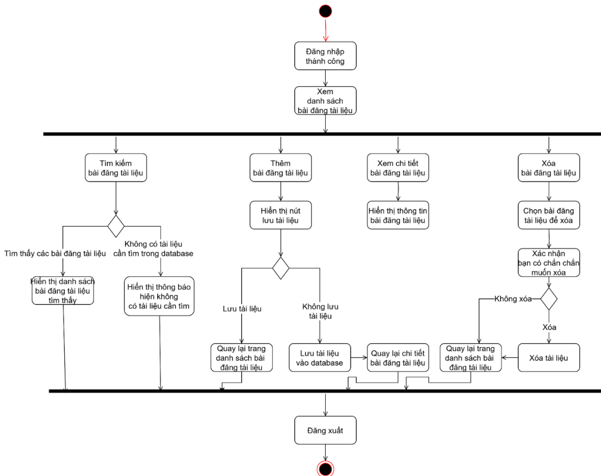
Hình 24: Activity diagram người dùng quản lý bài đăng
