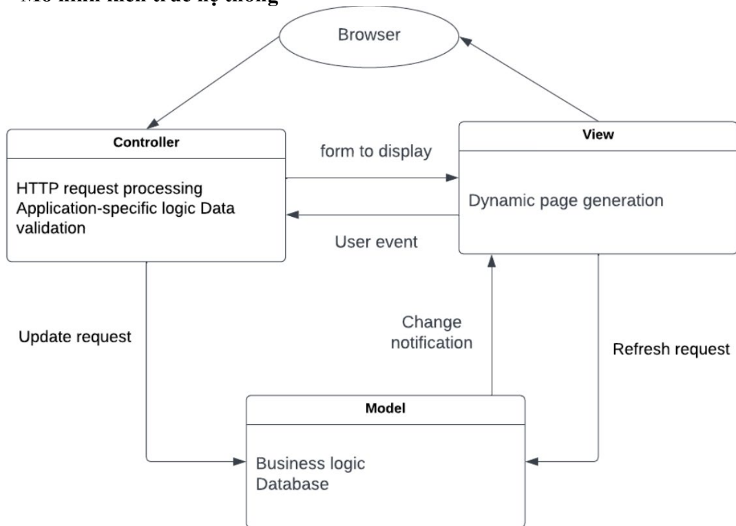
Hình 16: Mô hình kiến trúc hệ thống MVC
