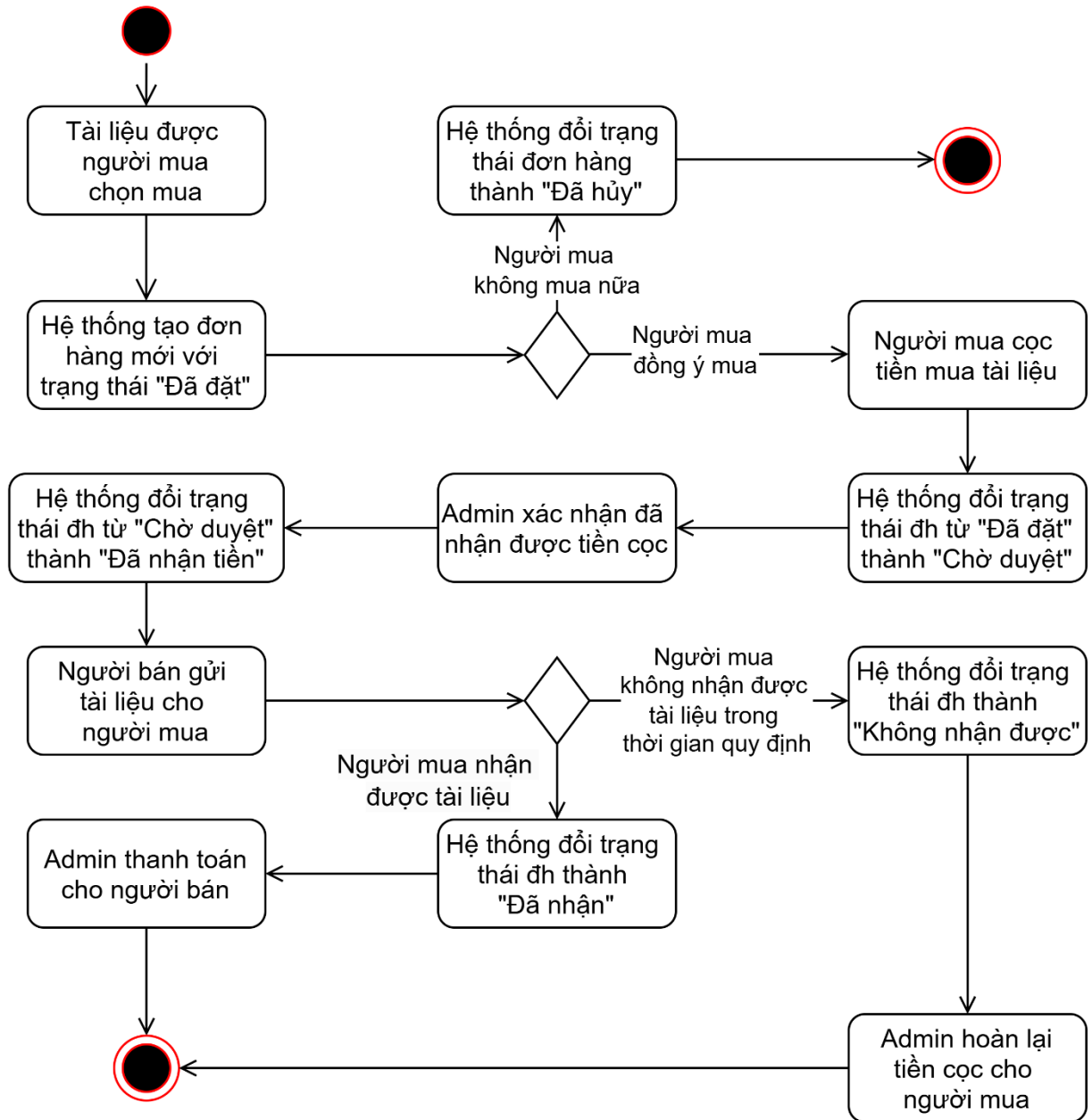
Hình 26: Activity diagram Người dùng mua tài liệu
