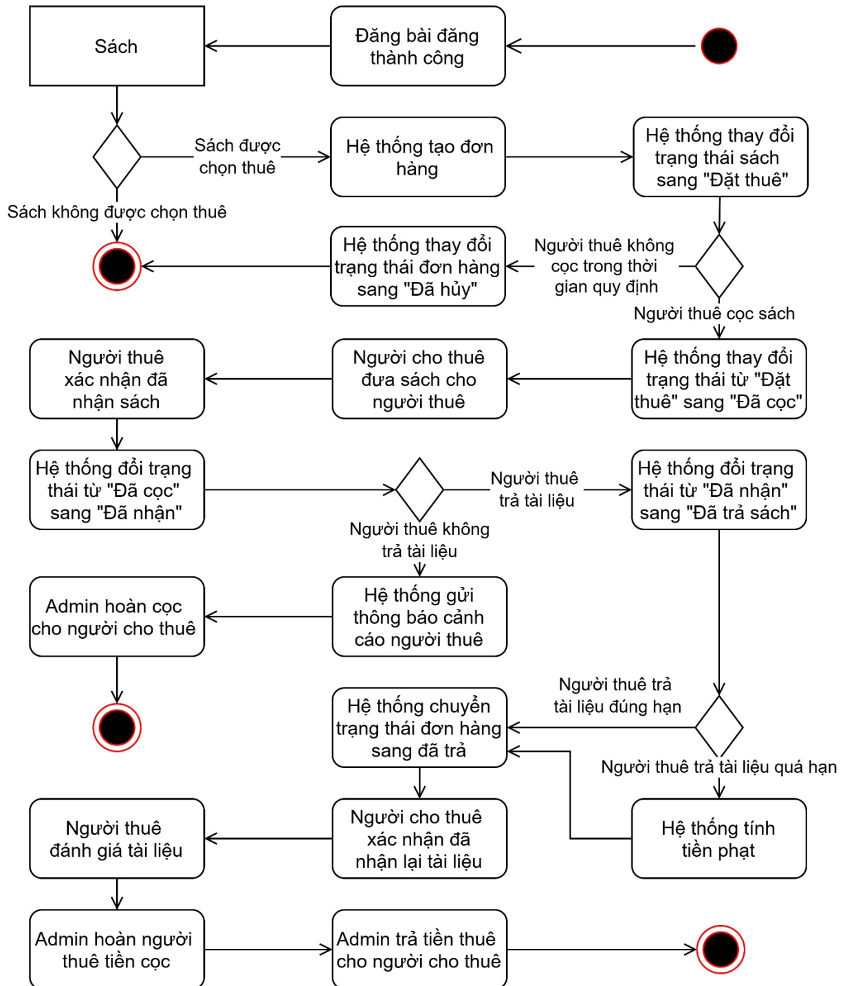
Hình 25: Activity diagram thuê và trả tài liệu
