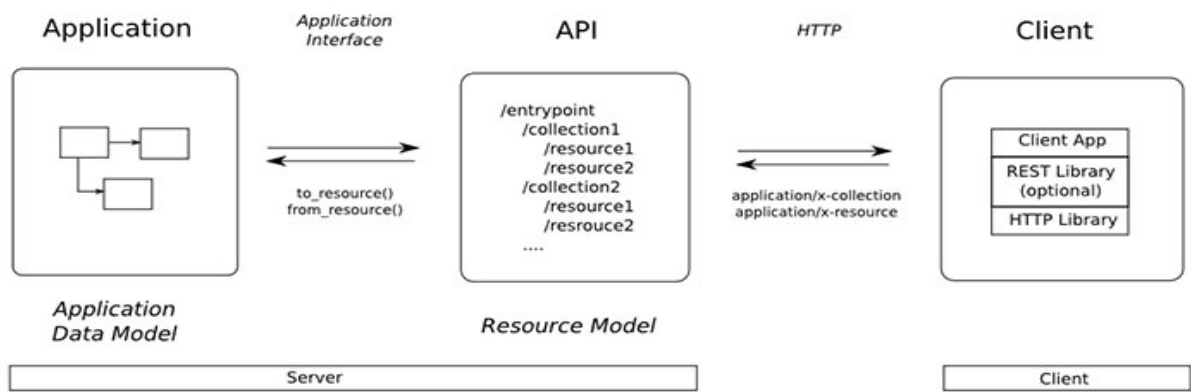
Hình 7: Nguyên tắc hoạt động của Restful API
