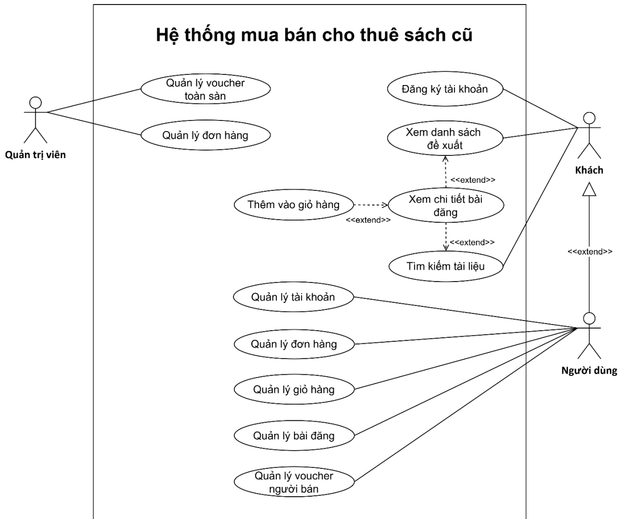
Hình 9: Use case diagram cho toàn bộ hệ thống
