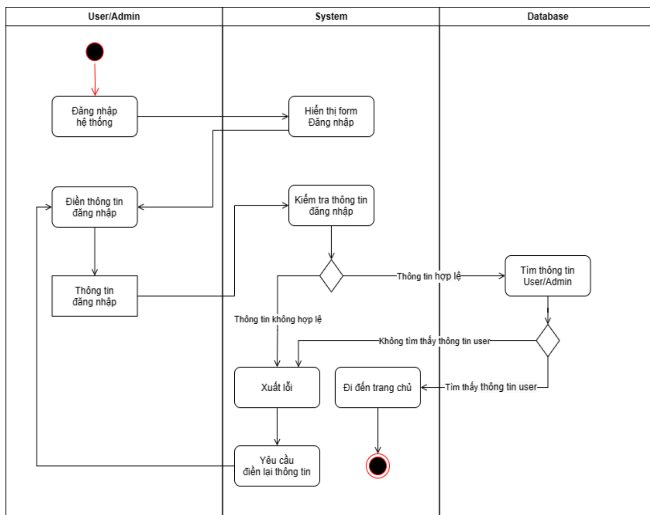
Hình 23: Activity diagram Quản trị viên và Người dùng với chức năng Đăng nhập
