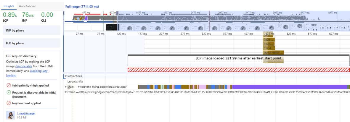
Hình 88: LCP Request Discovery
