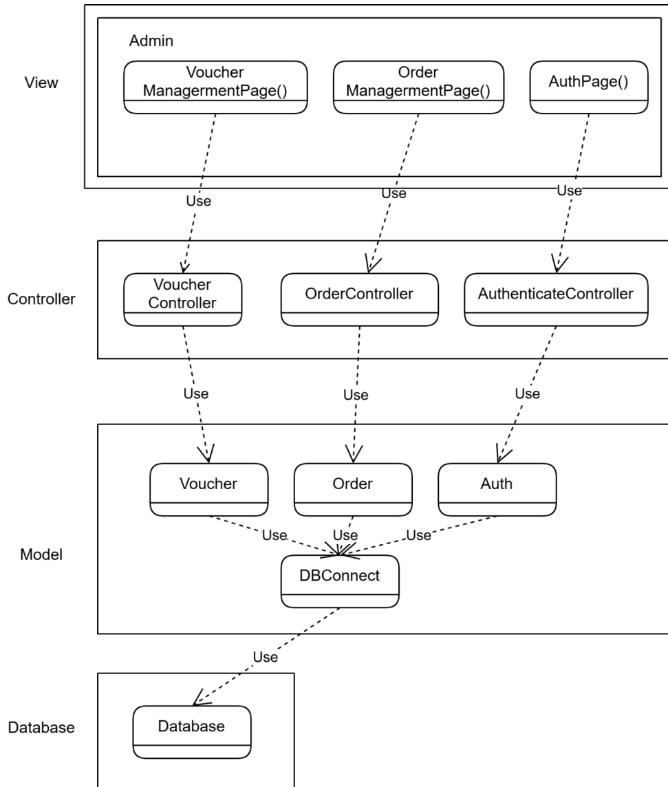
Hình 18: Layered architecture diagram cho quản trị viên
